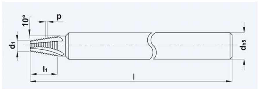
Kegel-Außen-Gewindfräser Conical external thread milling cutter
